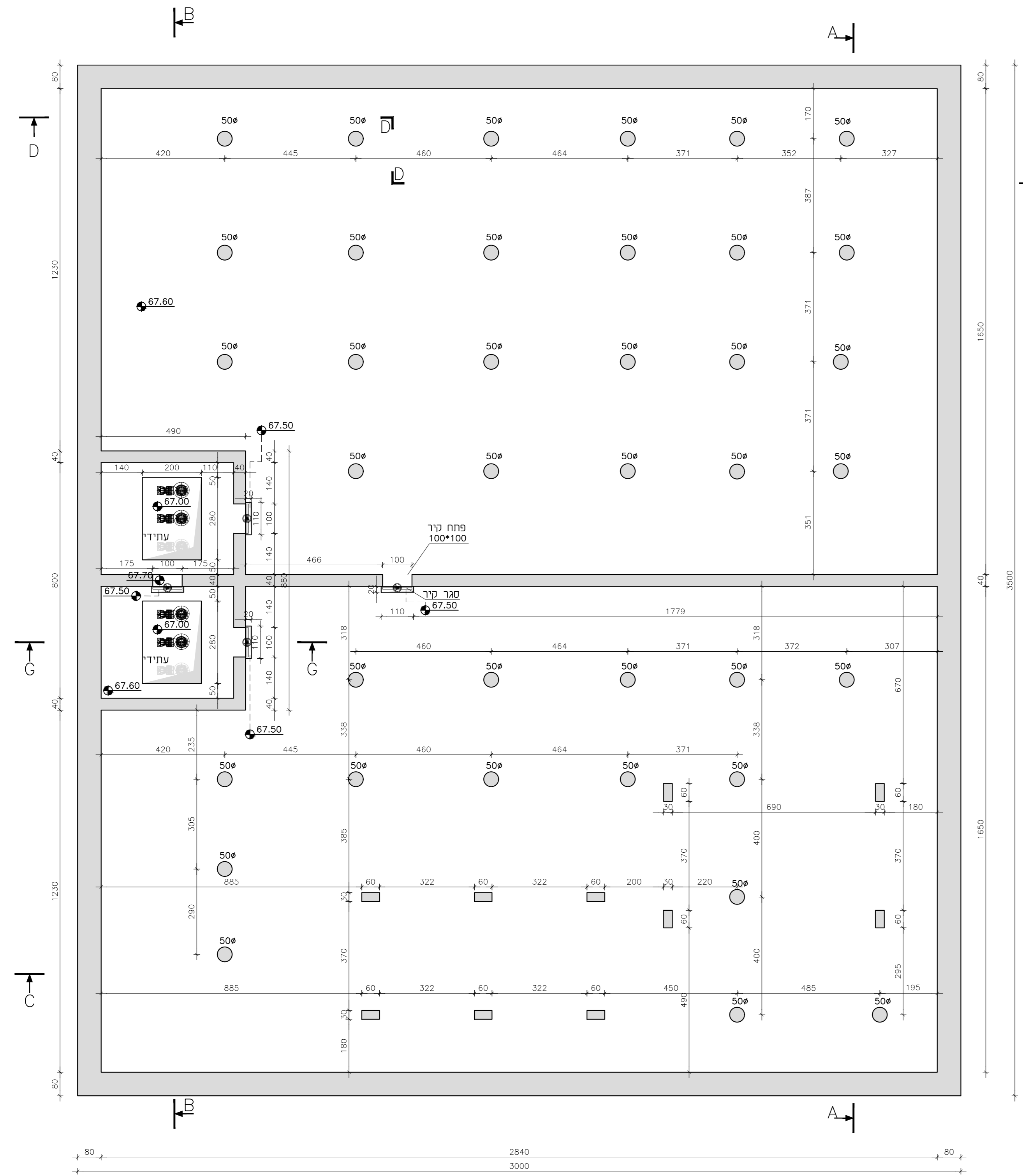
תכנית מפלס 67.80 קנ"מ: 1:100
